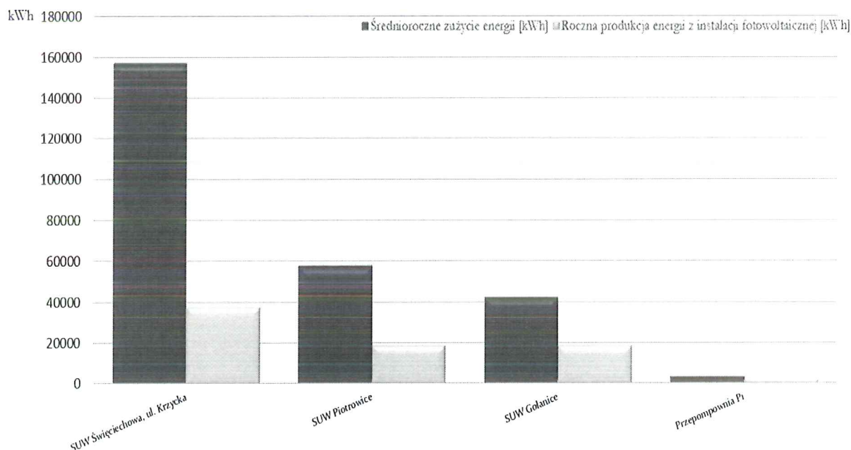
Rysunek nr 43. Zakładana produkcja energii elektrycznej w instalacjach PV przy infrastrukturze wod-kan
