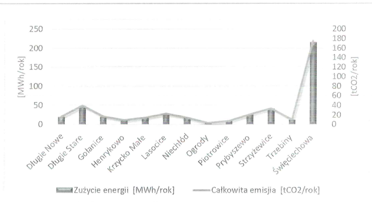
Rysunek nr 25. Łączne zużycie poszczególnych nośników energii wraz z produkcją CO 2 przez oświetlenie uliczne Źródło: Opracowanie własne
