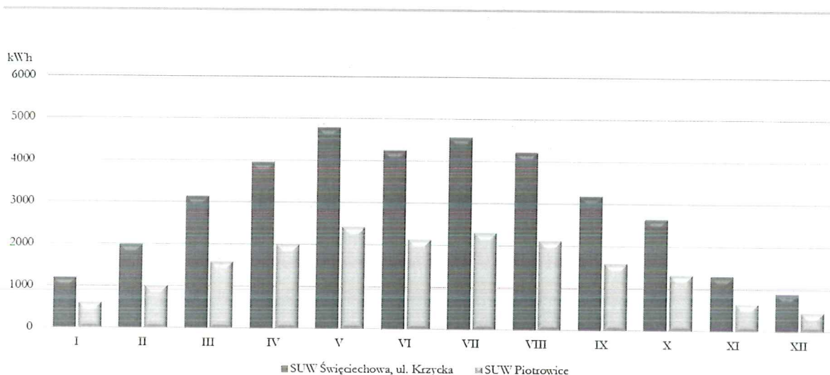
Rysunek nr 44. Zakładana produkcja energii elektrycznej w instalacjach PV przy infrastrukturze wod-kan Źródło: Opracowanie własne
