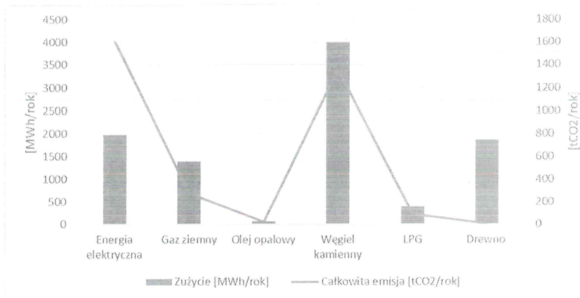
Rysunek nr 30. Łączne zużycie poszczególnych nośników energii wraz z produkcją CO 2 w budynkach usługowych
