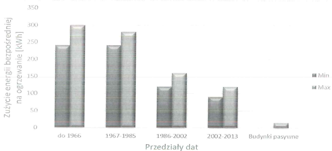
Rysunek nr 23. Wskaźnik zapotrzebowania na energię bezpośrednią na potrzeby ogrzewania wg roku oddania budynku do użytkowania Źródło: Opracowanie własne
