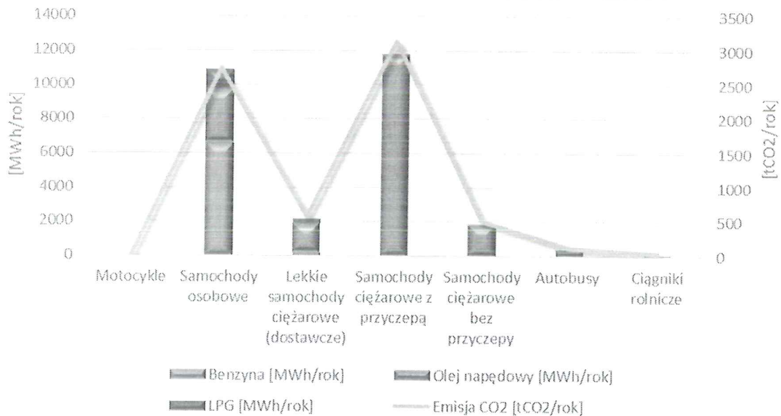
Rysunek nr 32. Łączne zużycie poszczególnych nośników energii wraz z produkcją CO 2 przez transport publiczny Źródło: Opracowanie własne
